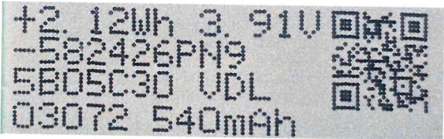
组成电池铭牌
