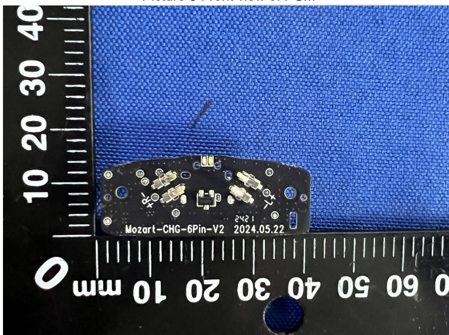
图 6 保护电路反面 Picture 6 Back view of PCM
