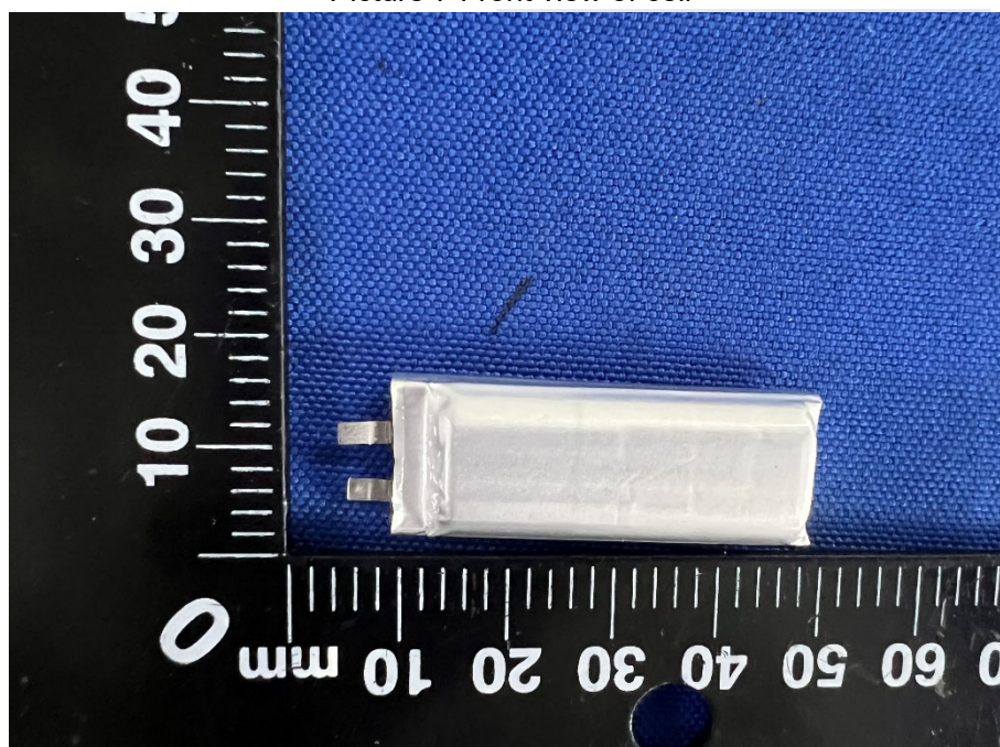
图 8 电芯背面
