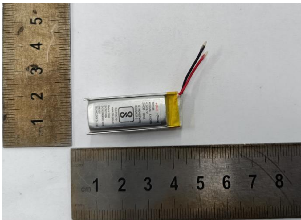
图 1 电芯正面 Picture 1 Front view of cell
