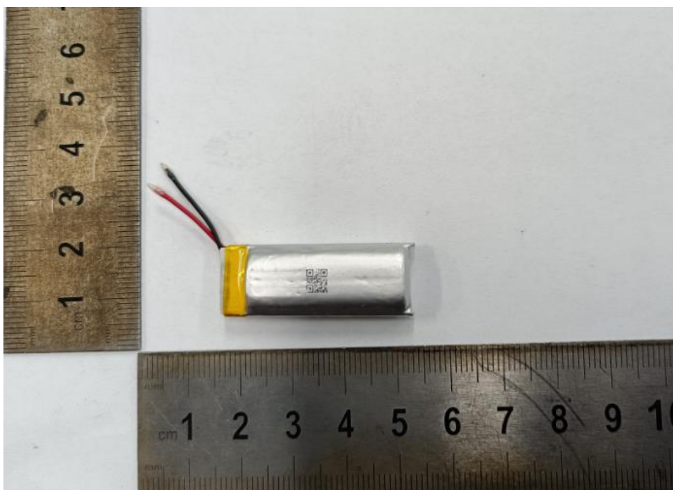
图 2 电芯反面 Picture 2 Back view of cell
